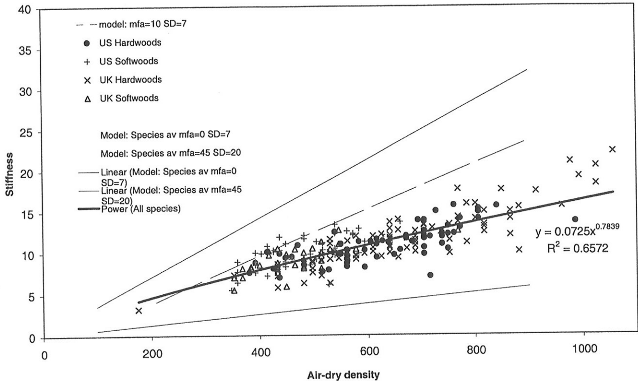
Abb. 7. Karte der Holzqualität, die den Dichteinfluss und die Ultrastruktur der Zellwand für alle Spezies enthält. Durchschnitt der gesamten Baumdaten. Die gepunkteten Linien zeigen theoretische Steifigkeitswerte an, die auf drei Größenbereichen der Mikrofibrillenwinkel basieren
