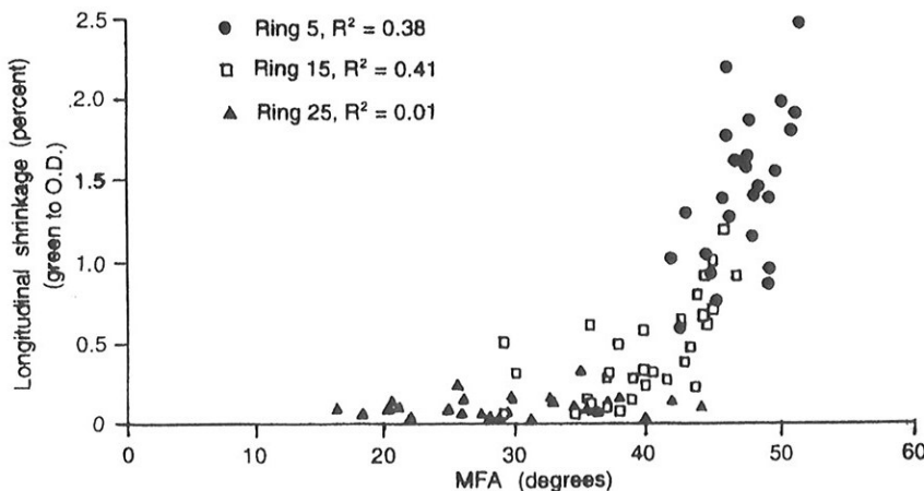
Fig. 10. Longitudinal shrinkage of loblolly pine as a function of microfibril angle for rings 5, 15 and 25 in butt samples of Pinus taeda (according to Megraw et al. 1998) Abb. 10. Längsschrumpfung von Loblollykiefer als Funktion des Mikrofibrillenwinkels für die Ringe 5, 15 und 25 in Endstammproben von Pinus taeda (nach Megraw et al. 1998)
