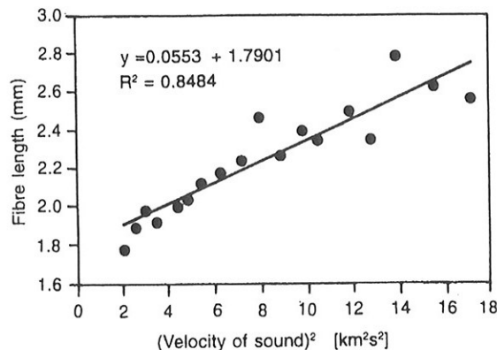
Fig. 21. Length-weighted average fiber length against the stress wave velocity in the logs (after NZ Patent 331527 1999) (Abb. 21. Längengewichtete Durchschnittsfaserlänge, aufgetragen gegen die Spannungswellengeschwindigkeit ins Rundholz (nach NZ Patent 331527 1999))
