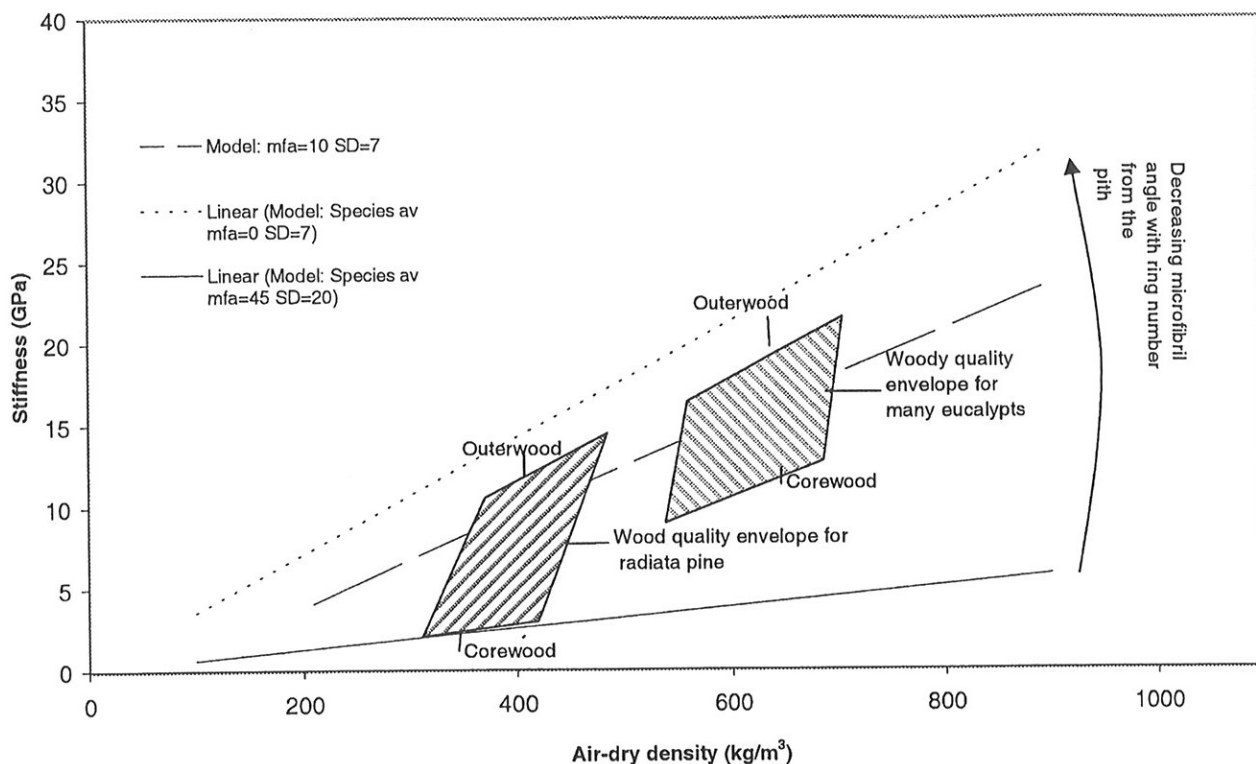
Abb. 8. Karte der Holzqualität, den Dichteinfluss und die Ultrastruktur der Zellwand für individuelle Reinholzproben von Pinus radiata und Eucalyptus nitens enthält—Daten innerhalb eines Baumes
