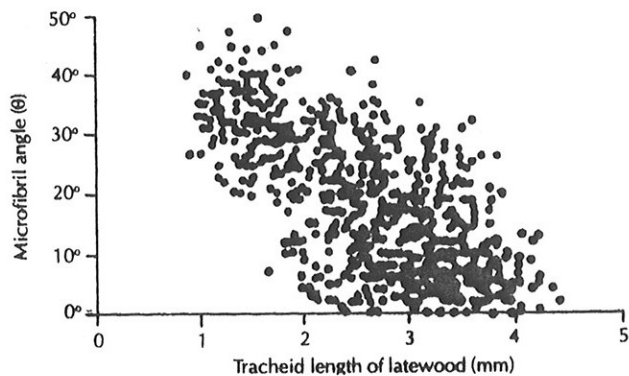
Fig. 20. Tracheid lengths and microfibril angles for macerated latewood tracheids of six clones using tissue from the 2nd, 6th, 16th and 20th growth rings (after Hirakawa, Fujisawa 1995) (Abb. 20. Tracheidenlängen und Mikrofibrillenwinkel für mazerierte Spätholztracheiden von sechs Klonen; verwendetes Gewebe von den 2., 6., 16. und 20. Jahresringen (nach Hirakawa, Fujisawa 1995))
