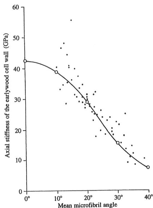
Fig. 4. The relationship between longitudinal Young's modulus and microfibril angle (experimental data) for Pinus radiata (according to Cave 1968) Abb. 4. Die Beziehung zwischen dem longitudinalen Youngs Modulus und dem Mikrofibrillenwinkel (experimentelle Daten) für Pinus radiata (nach Cave 1968)
