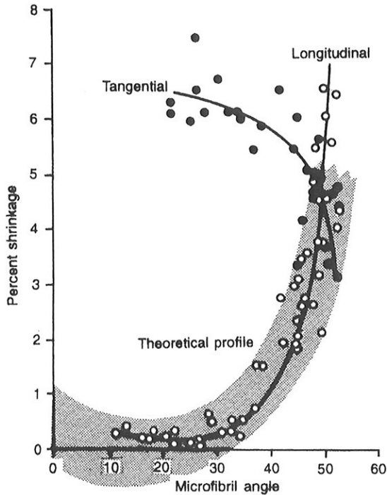
Fig. 9. Influence of microfibril angle on longitudinal shrinkage: experimental data for Pinus jeffreyi discs from breast height (after Meylan 1968), on which has been superimposed a band of theoretical profiles, depending on the stiffness and shear modulus of the cellulose and hemicelluloses-lignin matrix, respectively (adapted from Barber, Meylan 1964) Abb. 9. Einfluss des Mikrofibrillenwinkels auf die Längsschrumpfung: experimentelle Daten für Pinus jeffreyi Scheiben in Brusthöhe (nach Meylan 1968), über das ein Band theoretischer Profile überlagert wurde, je nach Steifigkeit bzw. der Scherfestigkeit der Cellulosen- und Hemicellulosen-Lignin-Matrix. (angepasst nach Barber, Meylan 1964)
