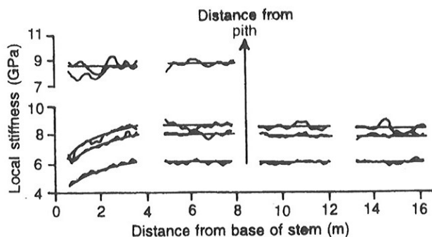
Fig. 15. Radial and axial variations in the mean local bending stiffness of sawn lumber cut from the same logs as in Fig. 13 (according to Xu and Walker, in press) Abb. 15. Radiale und axiale Variationen in der mittleren lokalen Biegesteifigkeit von Schnittholz, aus dem gleichen Rundholz wie in Abb. 13 (nach Xu und Walker, im Druck)
