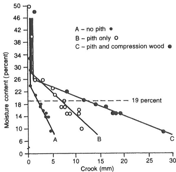
Fig. 11. Crook, arising from excessive shrinking along one edge of the board, is more prevalent in lumber cut to include the pith or with compression wood (modified from Gaby 1972) Abb. 11. Eine Krümmung, die von exzessiver Schrumpfung entlang der Brettkante herrührt, ist häufiger in Schnittholz mit Mark und Druckholzanteilen vorhanden (modifiziert von Gaby 1972)
